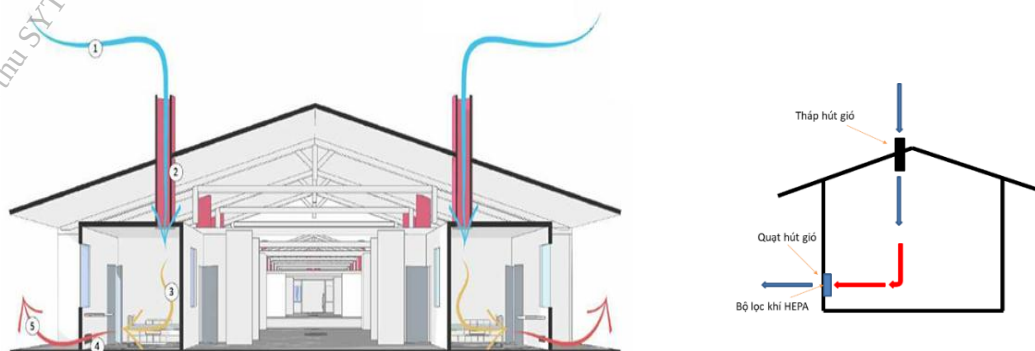
Hình 9. Mô hình thông khí phối hợp và sơ đồ xử lý khí thải
